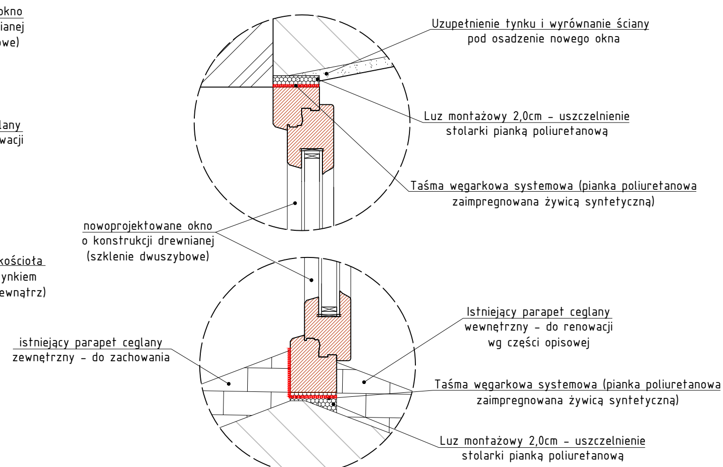
DETALE MONTAŻU
