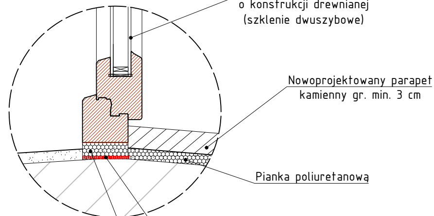
Luz montażowy 2,0cm - uszczelnienie stolarki pianką poliuretanową
