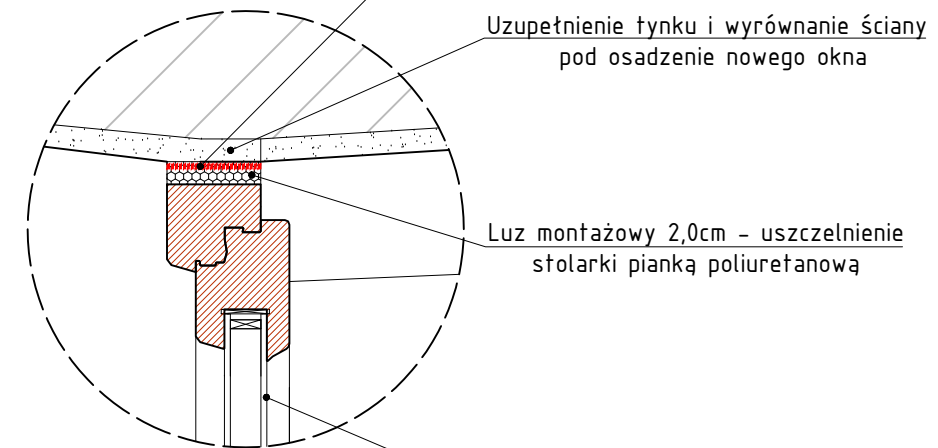
nowoprojektowane okno o konstrukcji drewnianej (szklenie dwuszybowe)
