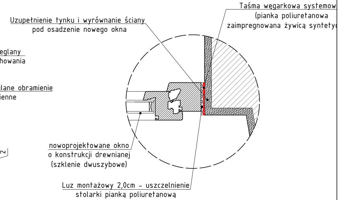
DETALE MONTAŻU
