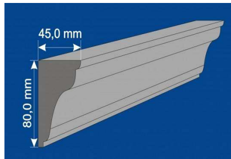
Przykładowy przekrój gzymsu parapetowego.
