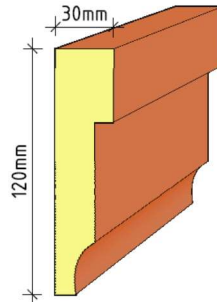
Przykładowy przekrój przez opaskę okienną.
